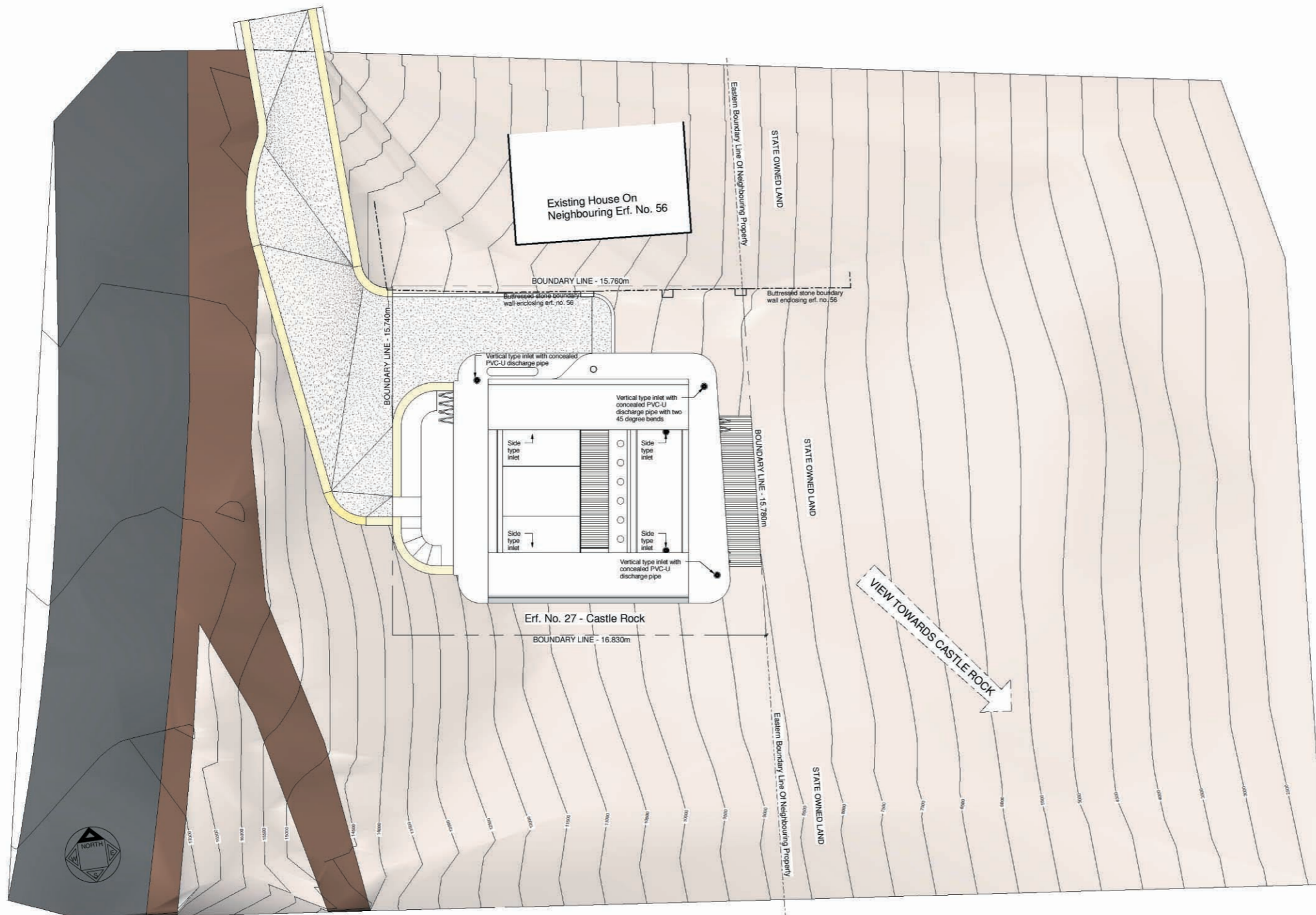
SITE PLAN 1 : 100
