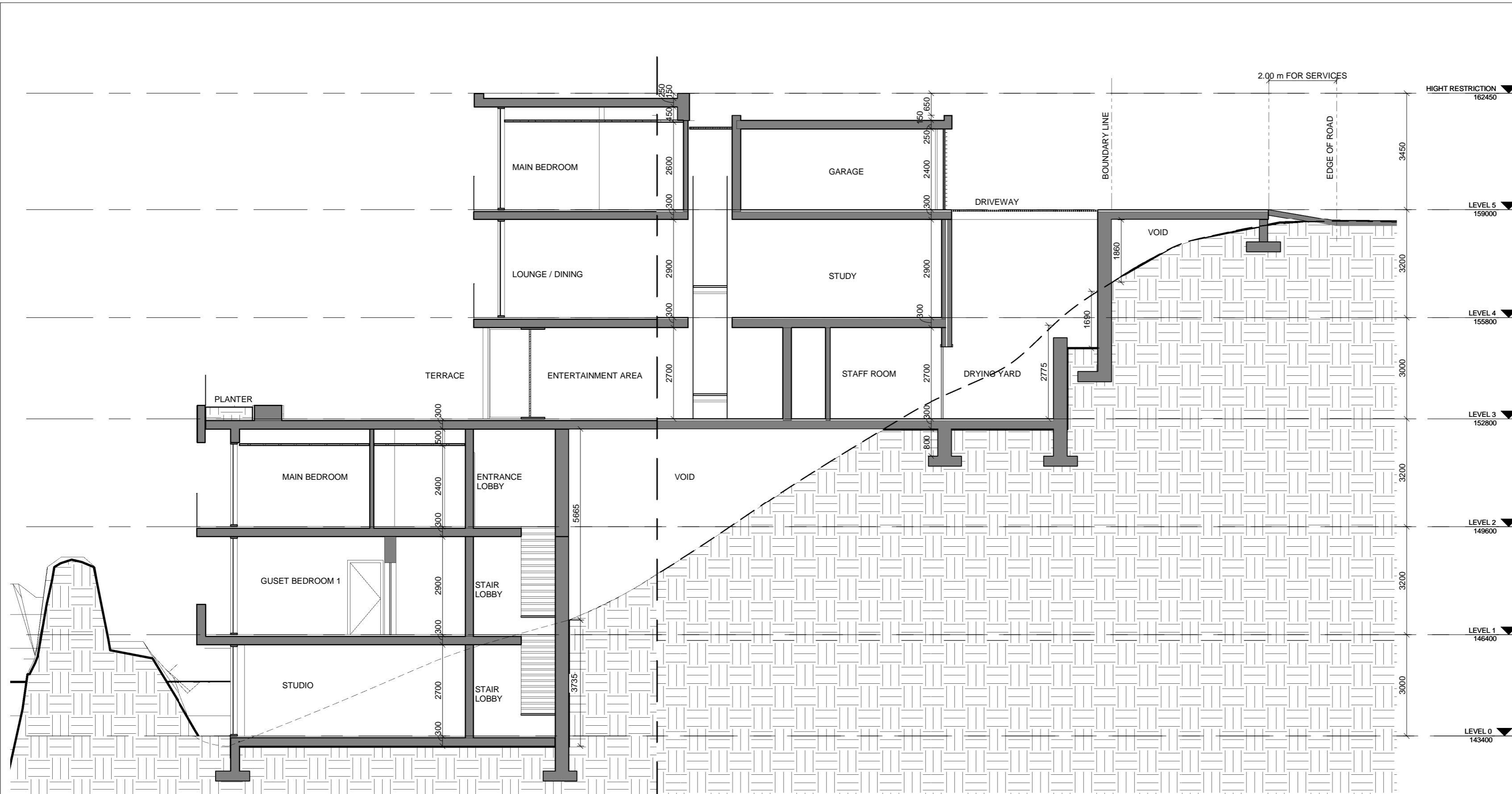
SECTION D 1 1 : 100
